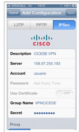
Figura 6. Parámetros de configuración de VPN IPSec.
